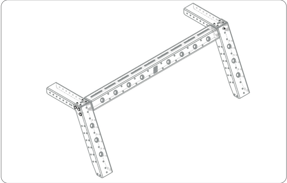
Abb. 4: komplett verschraubte Eckstrebe / completely bolted corner strut
